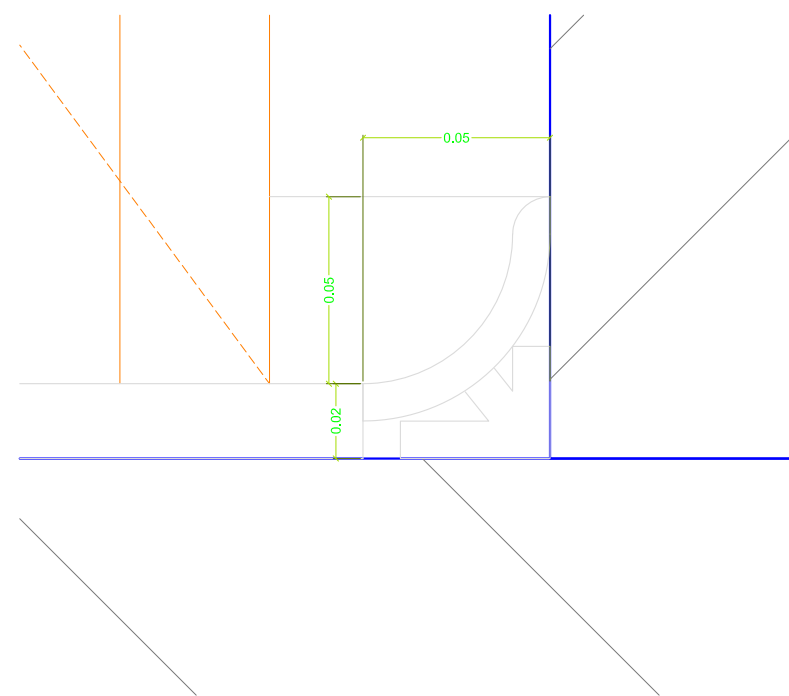
DETALLE MEDIACAÑA 5CM X 5CM ESC: 1:2
