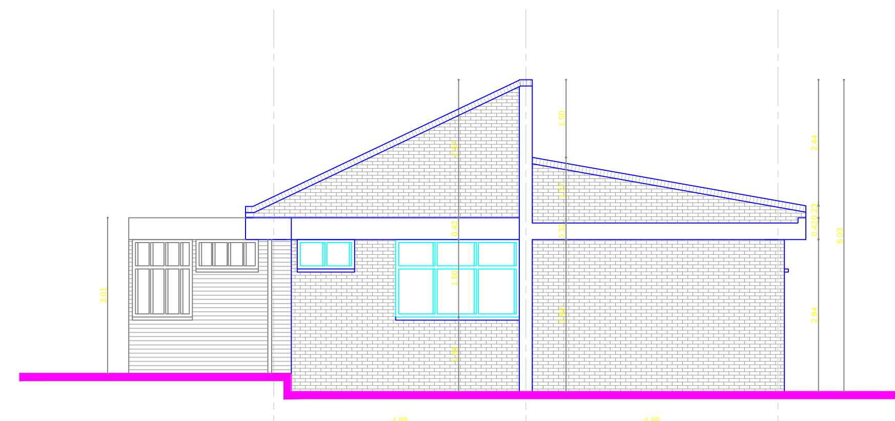
FACHADA ORIENTAL
