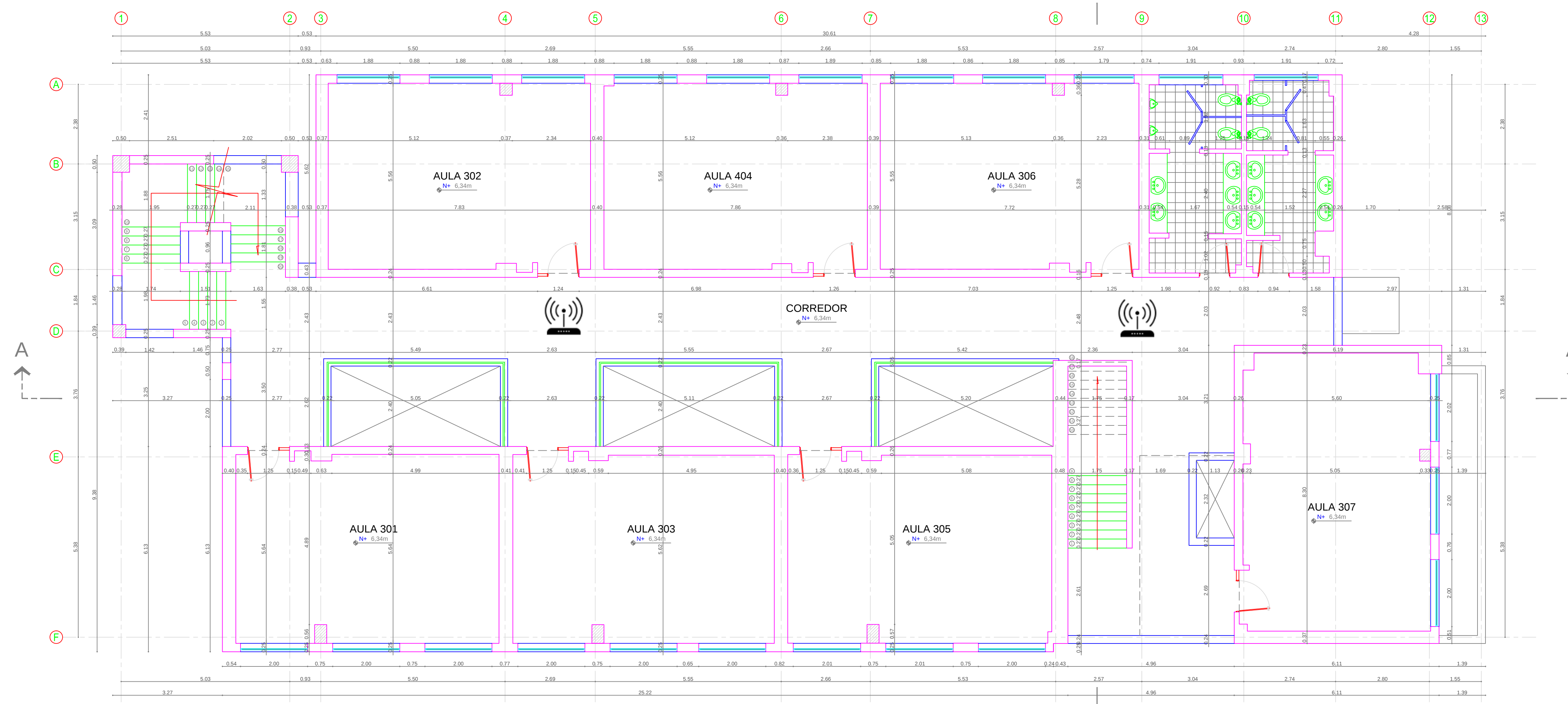
PLANTA TERCER PISO
