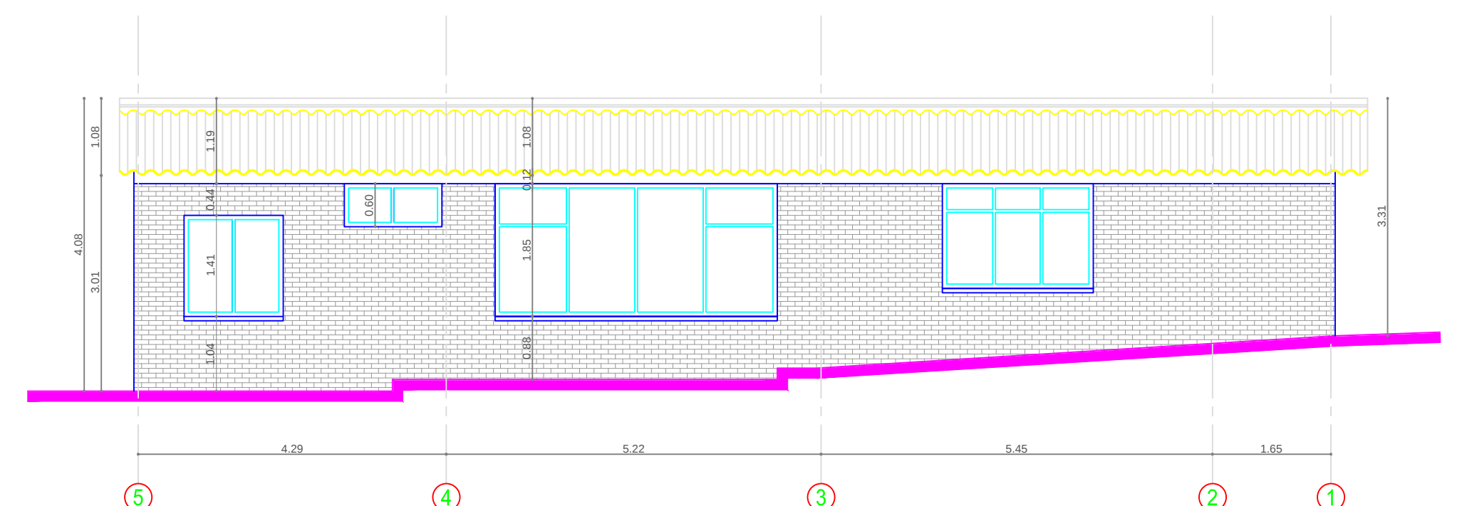
FACHADA SUR
