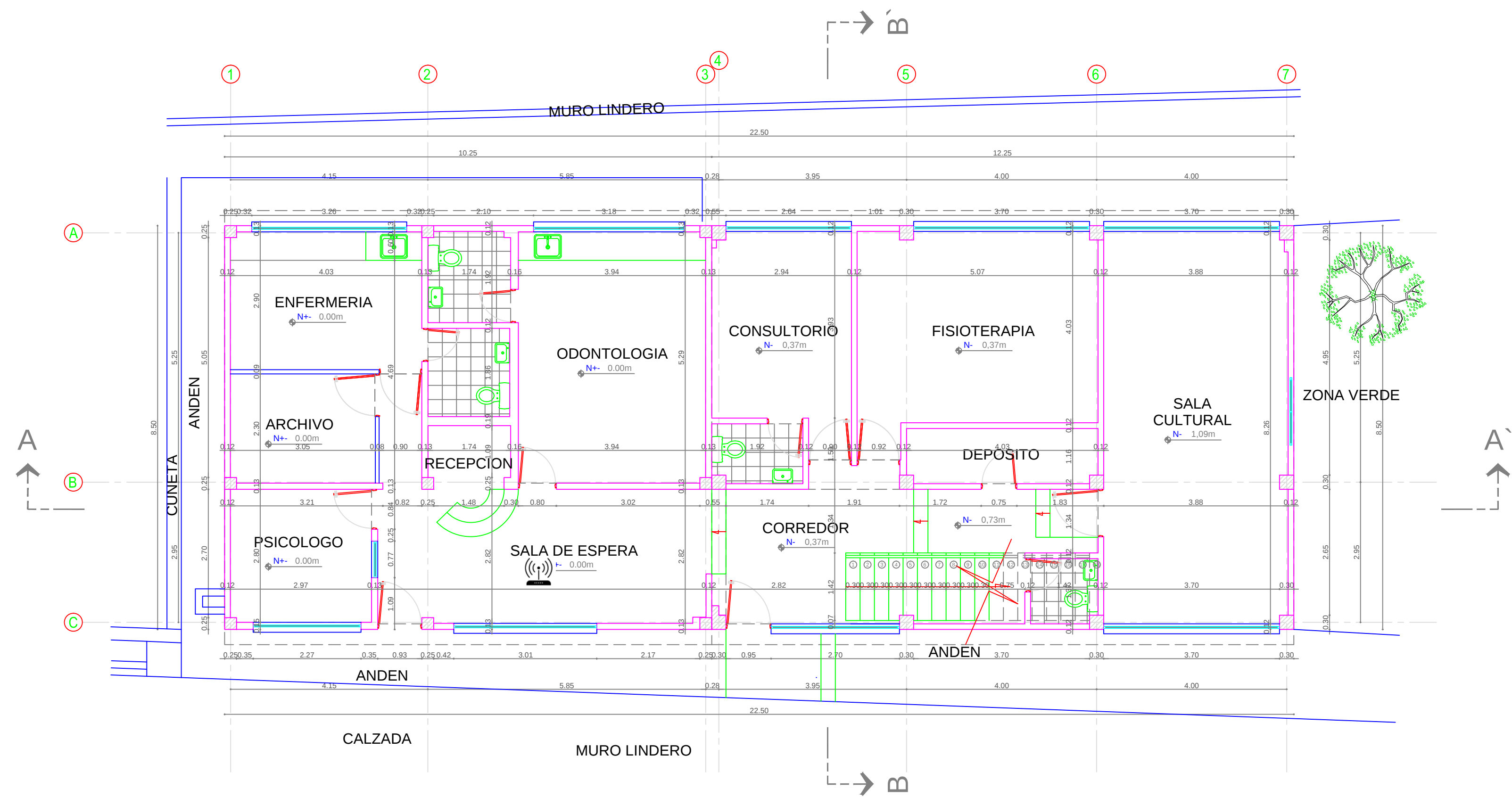
PLANTA PRIMER PISO
