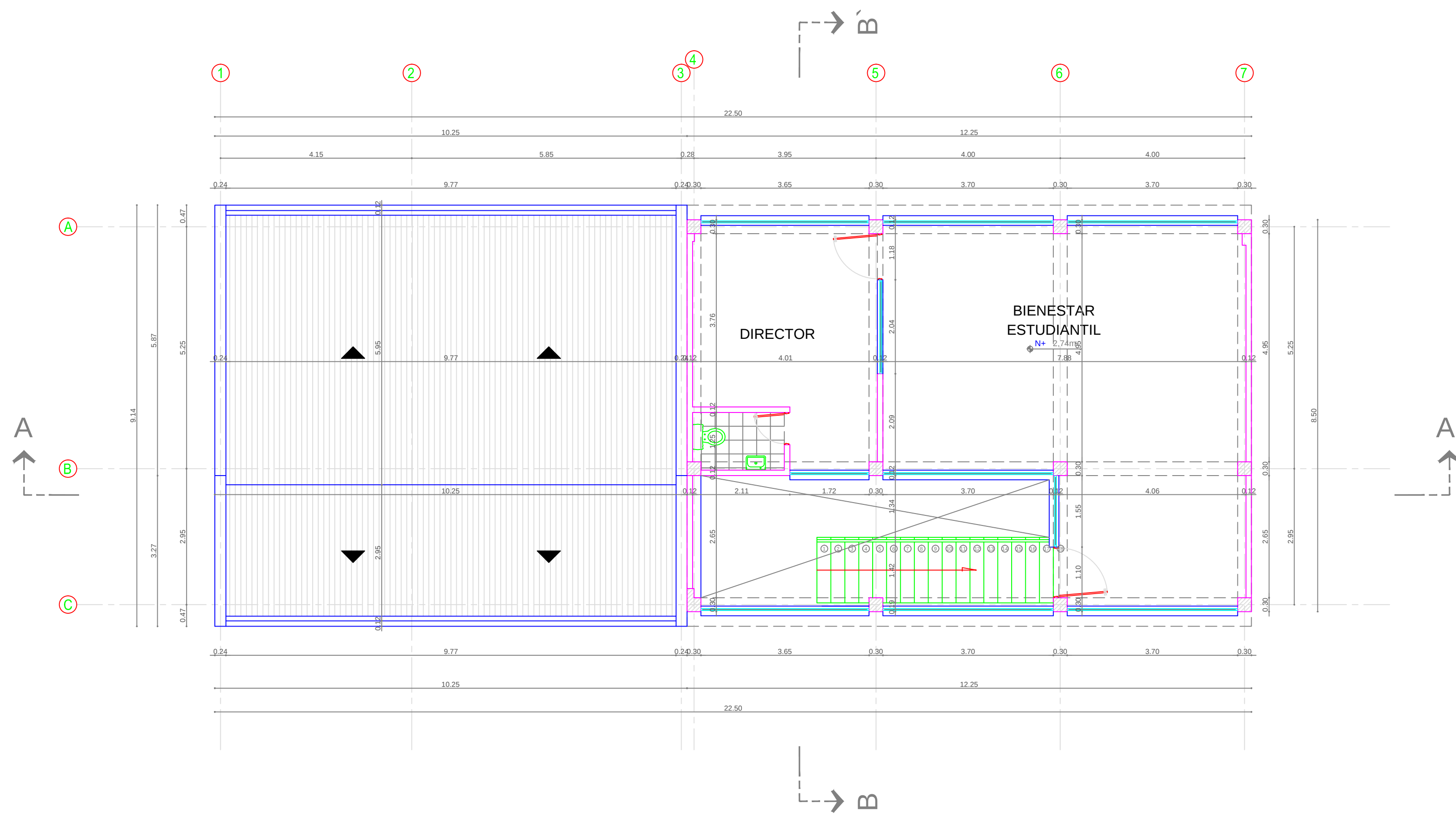
PLANTA SEGUNDO PISO
