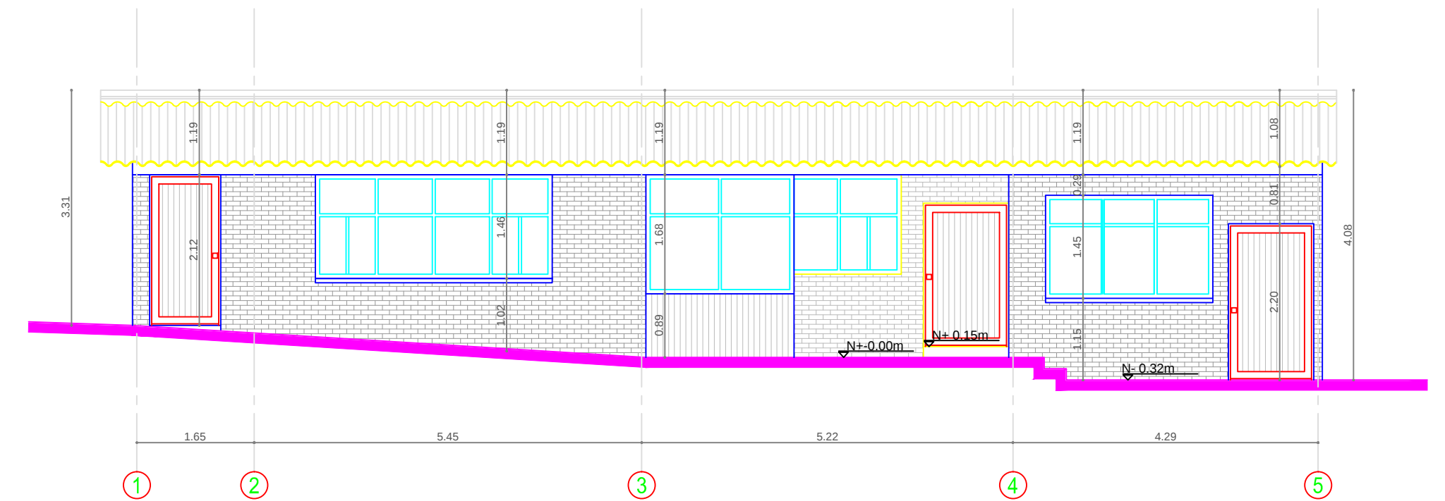
FACHADA NORTE
