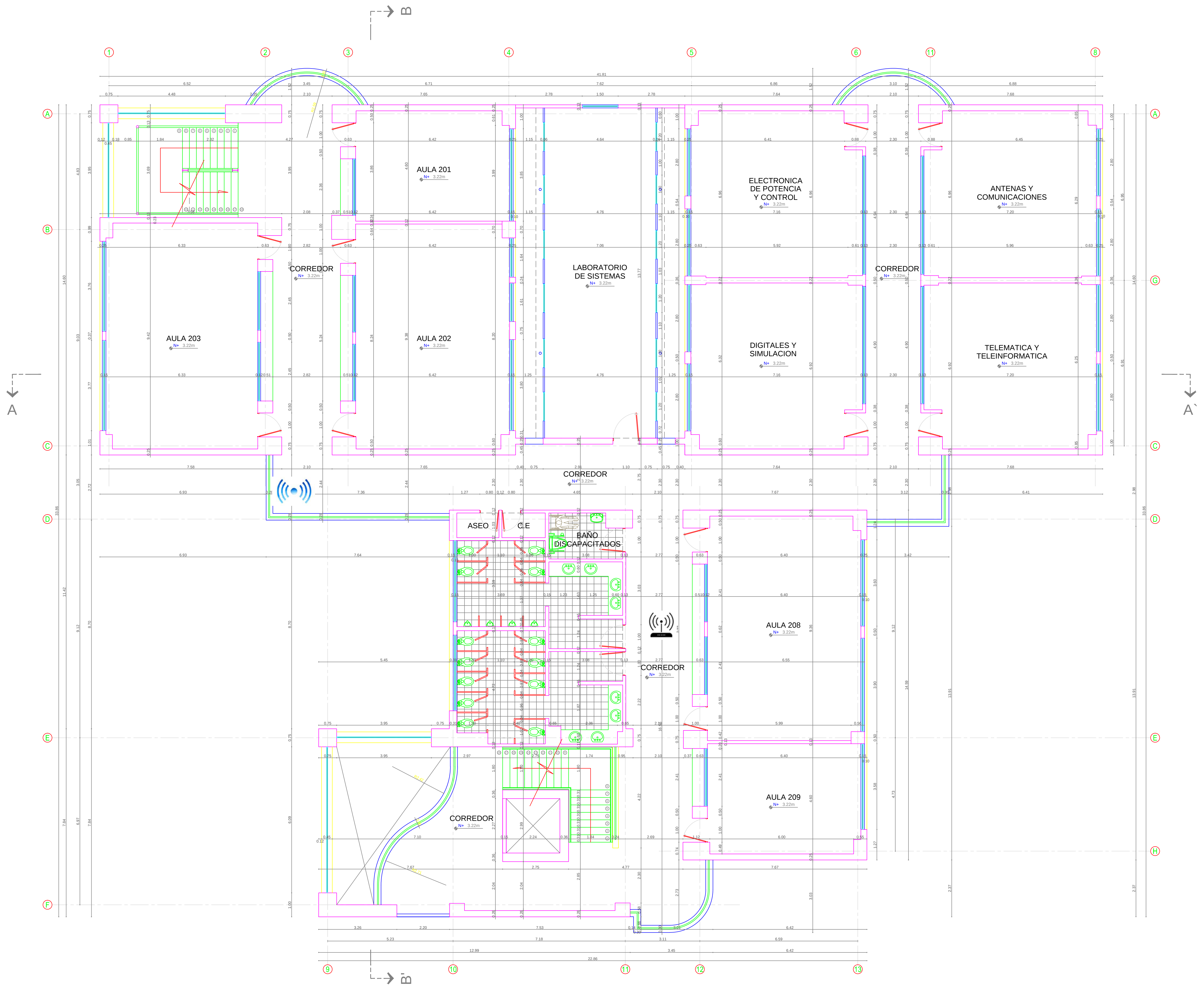
PLANTA SEGUNDO PISO BLOQUE F
