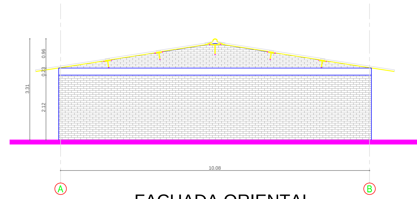
FACHADA ORIENTAL
