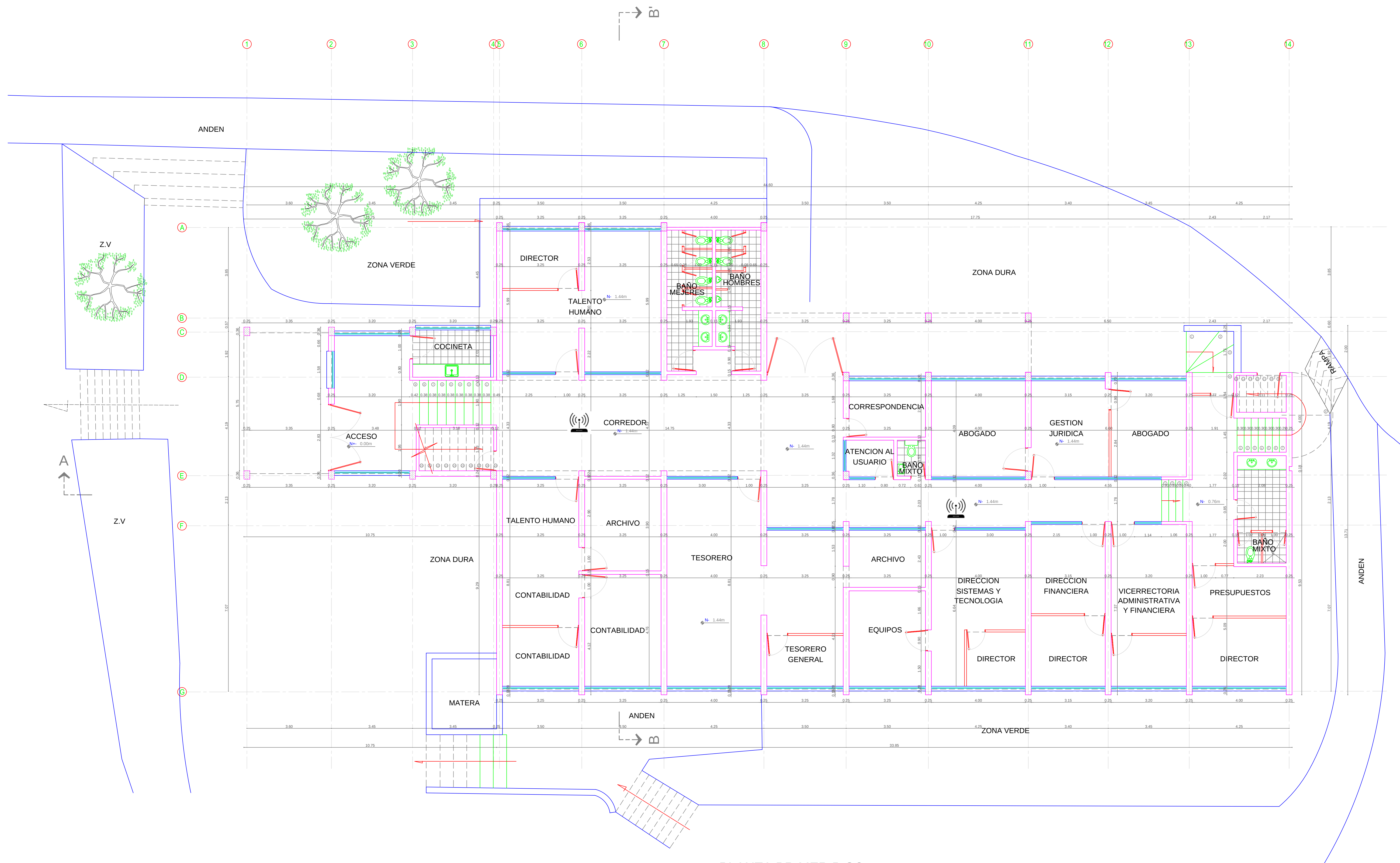
PLANTA PRIMER PISO
