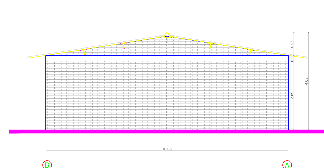
FACHADA OCCIDENTAL
