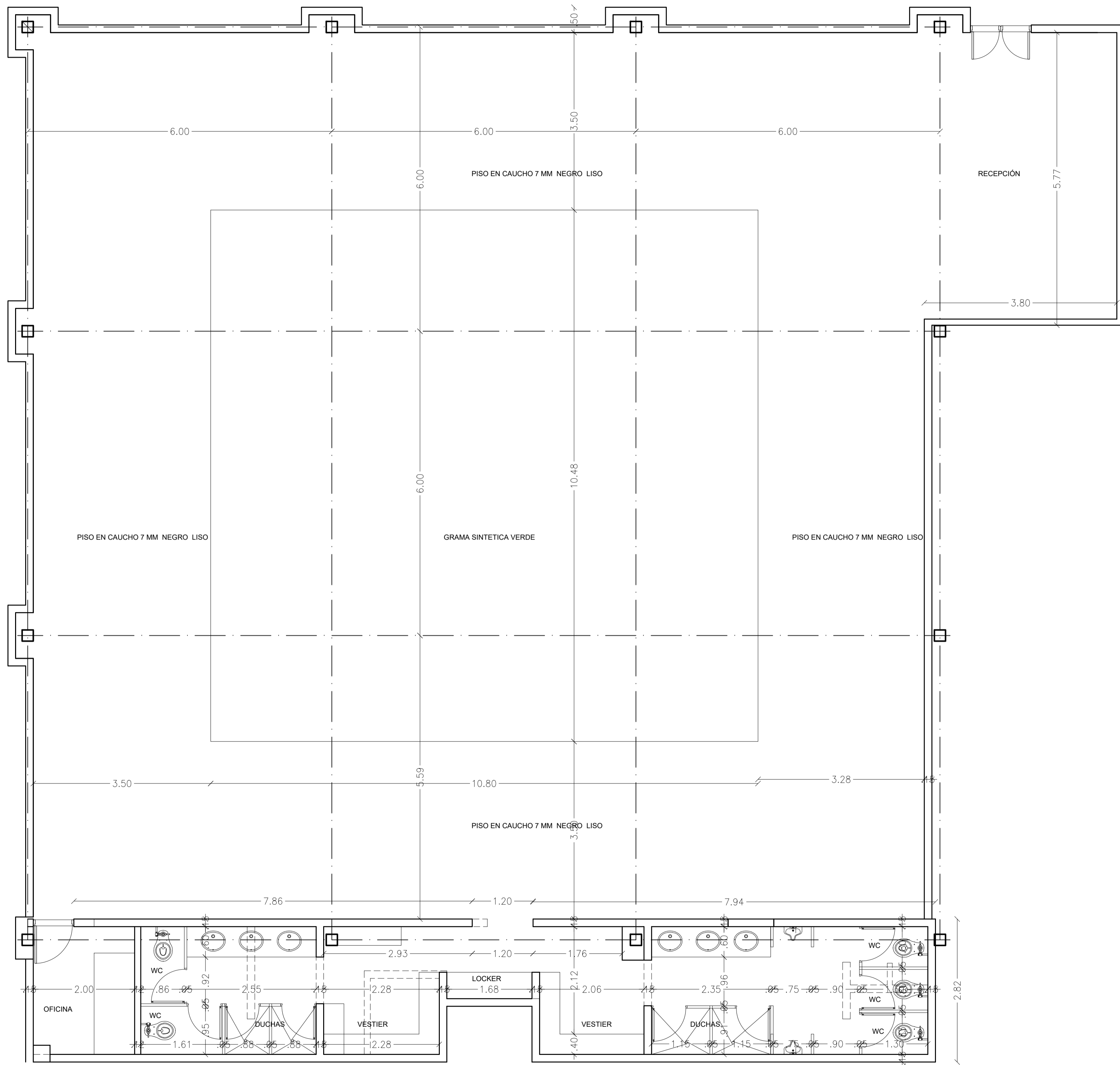
PLANTA ARQUITECTONICA ZONA GIMNASIO ESC: 1:50
