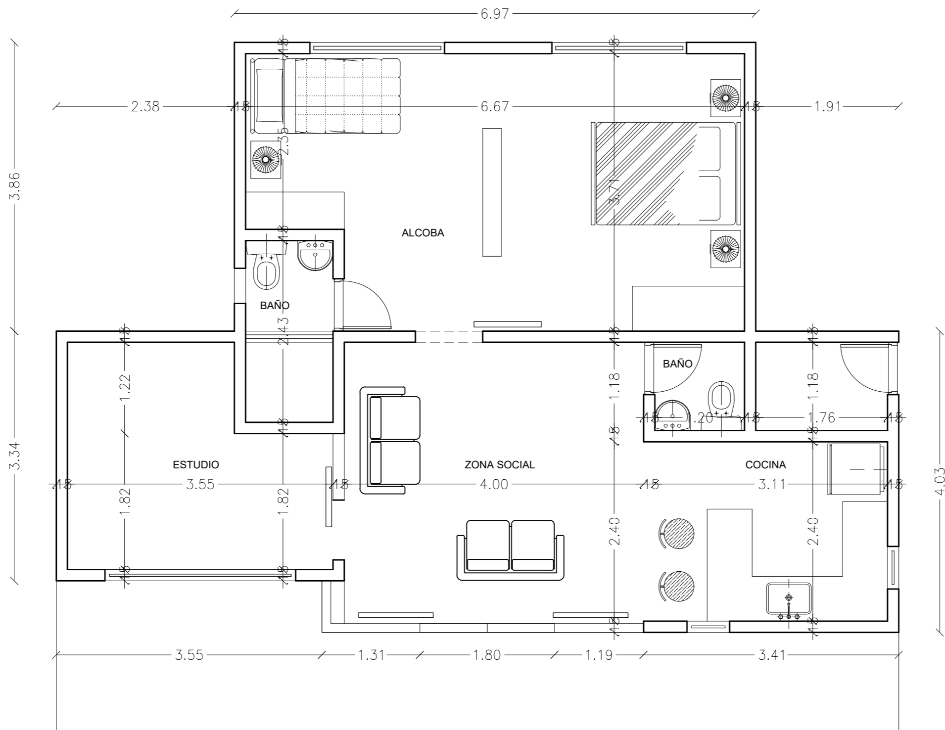
PLANTA ARQUITECTONICA CABAÑA ESC: 1:50
