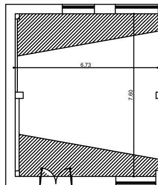
PLANTA ARQUITECTÓNICA
