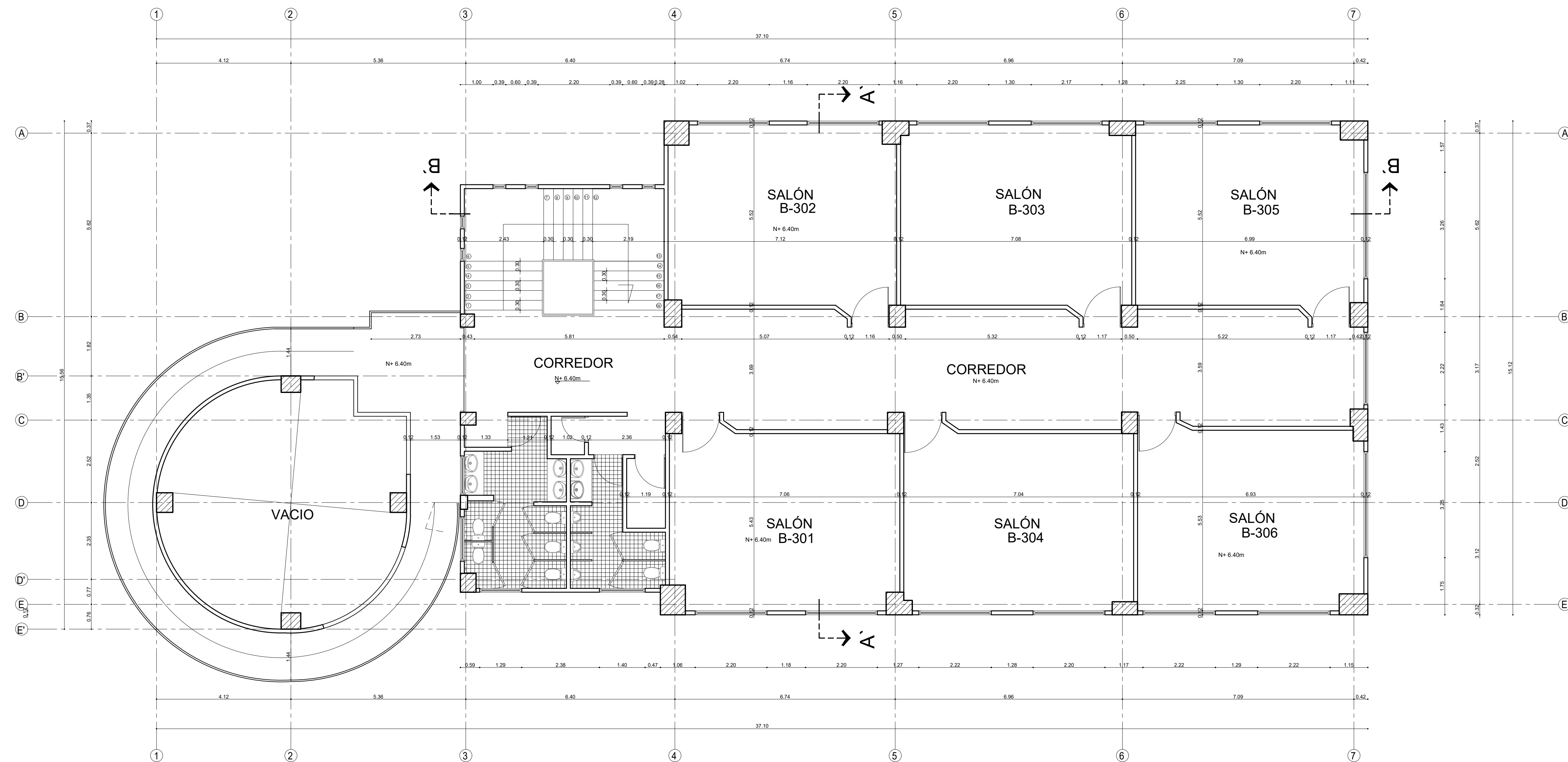
PLANTA TERCER PISO
