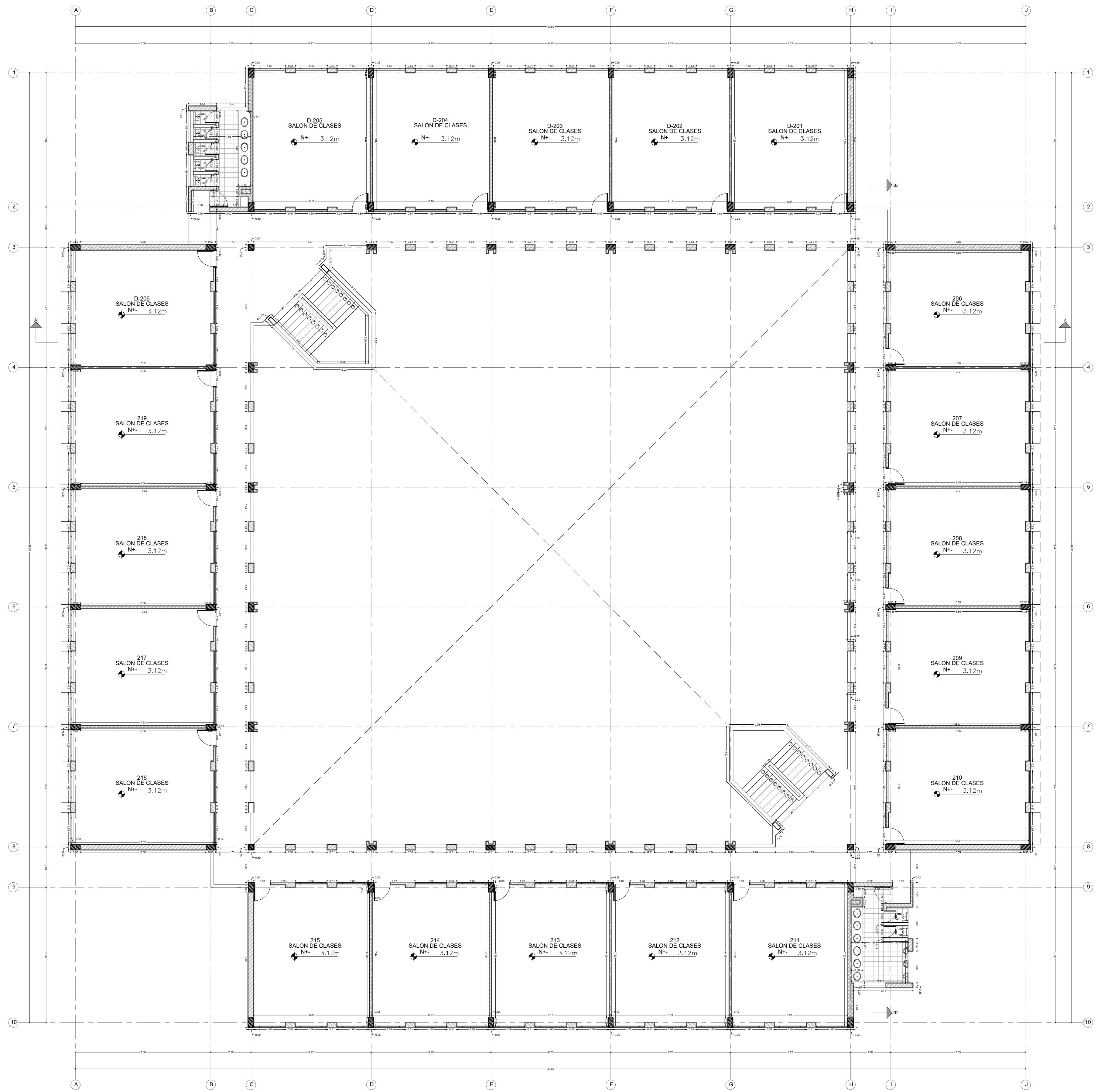
PLANTA SEGUNDO PISO
