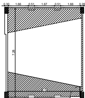
PLANTA ARQUITECTÓNICA
