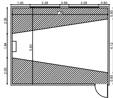
PLANTA ARQUITECTÓNICA
