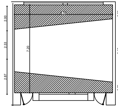
PLANTA ARQUITECTÓNICA
