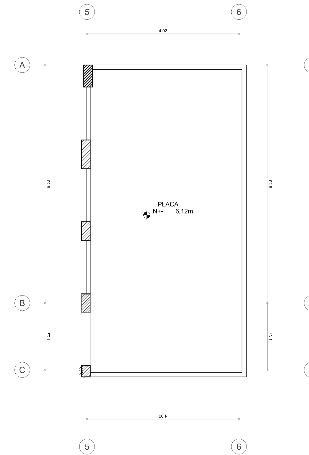
PLANTA CUBIERTAS
