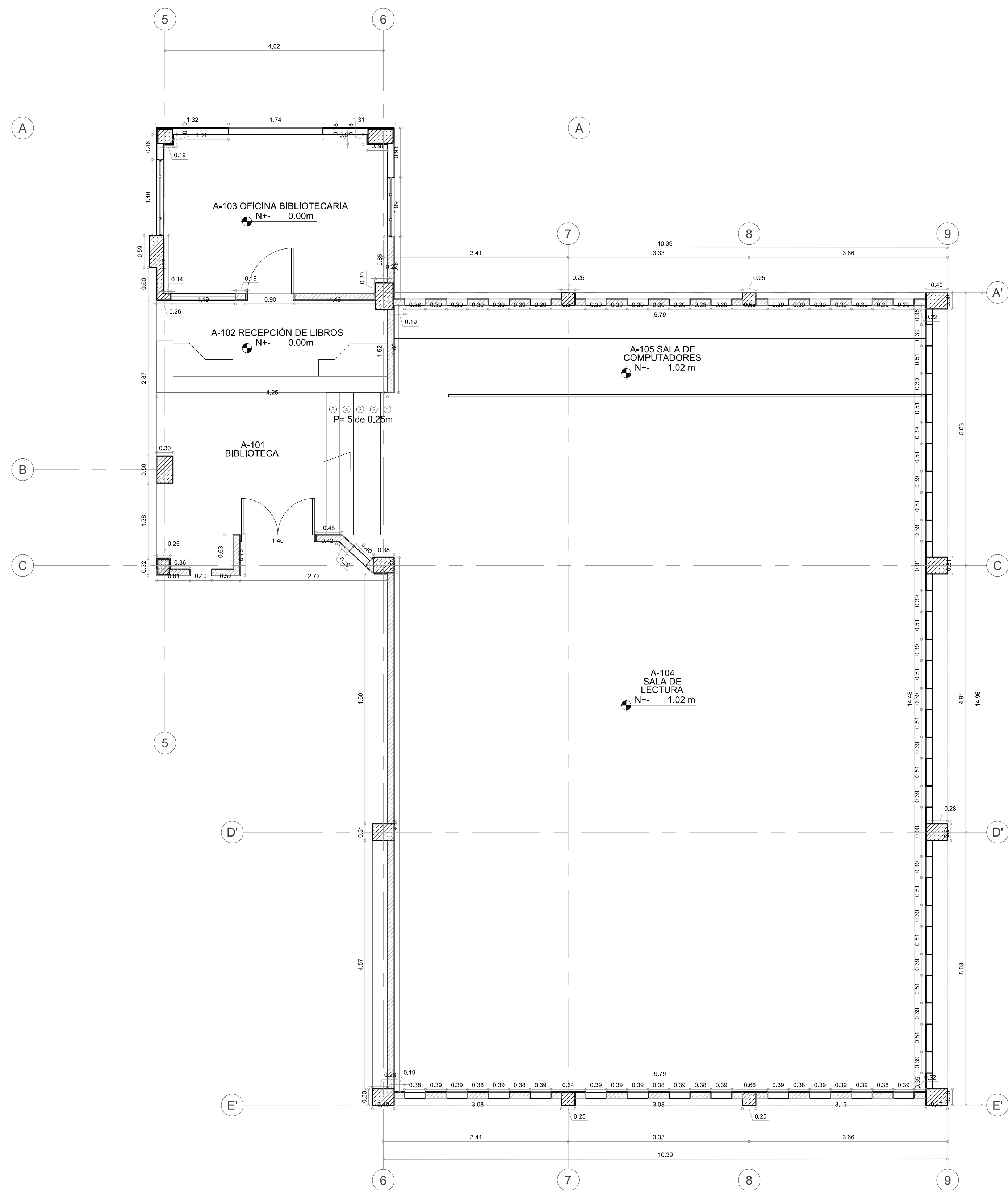
PLANTA PRIMER PISO ACTUAL
