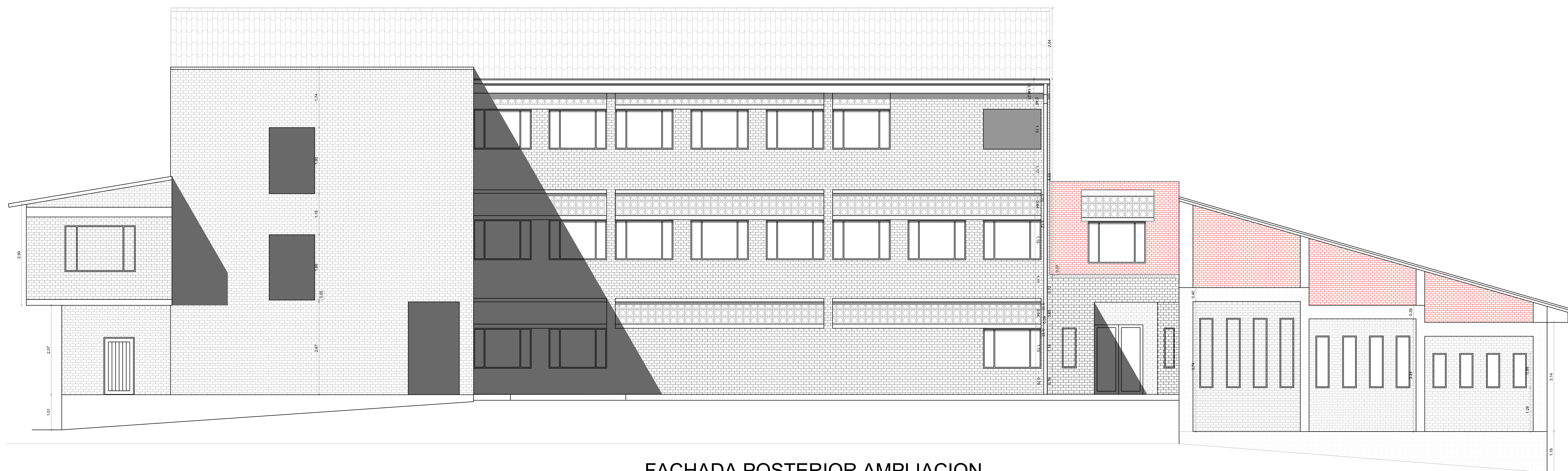
FACHADA POSTERIOR ACTUAL
