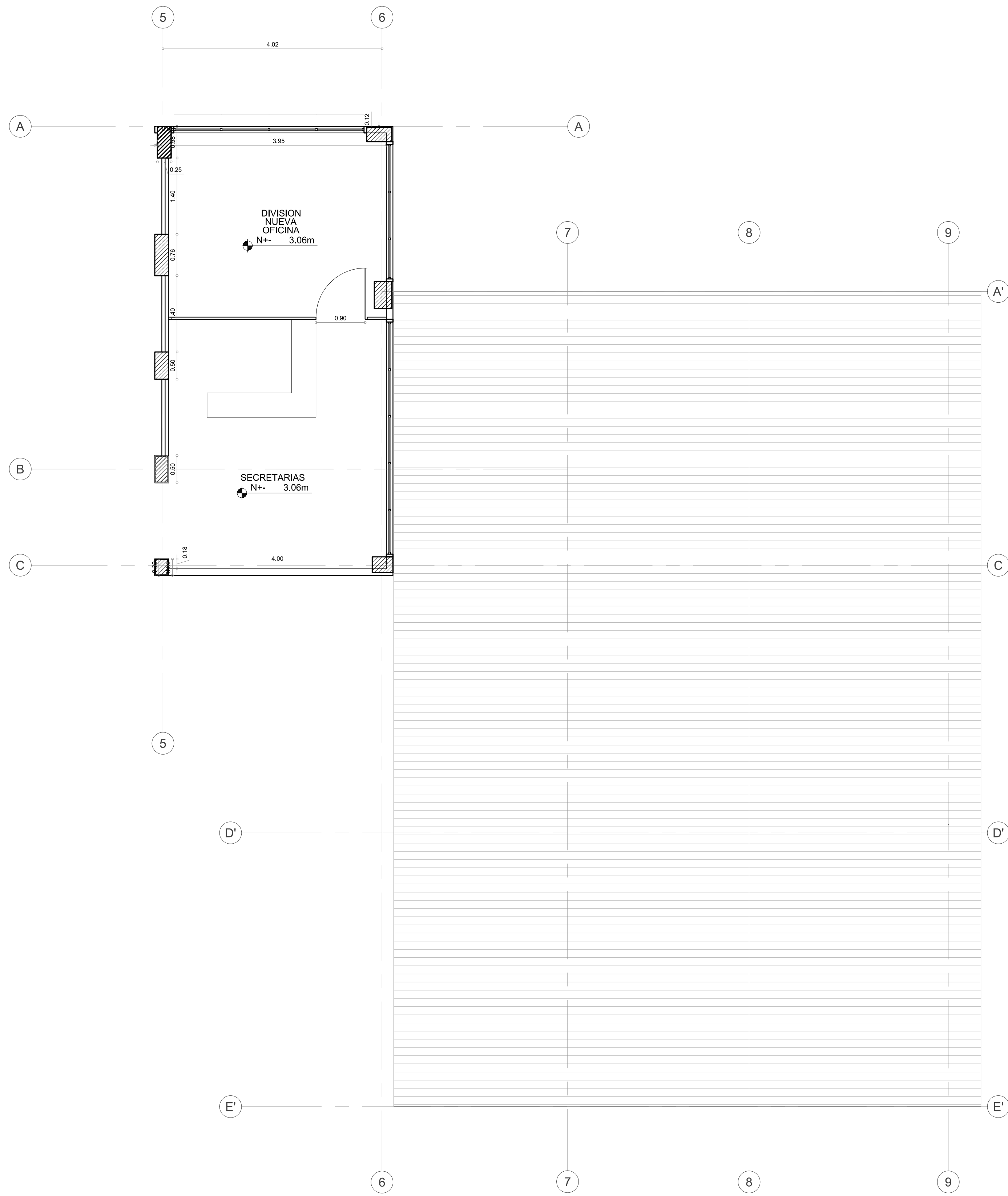
PLANTA SEGUNDO PISO AMPLIACION
