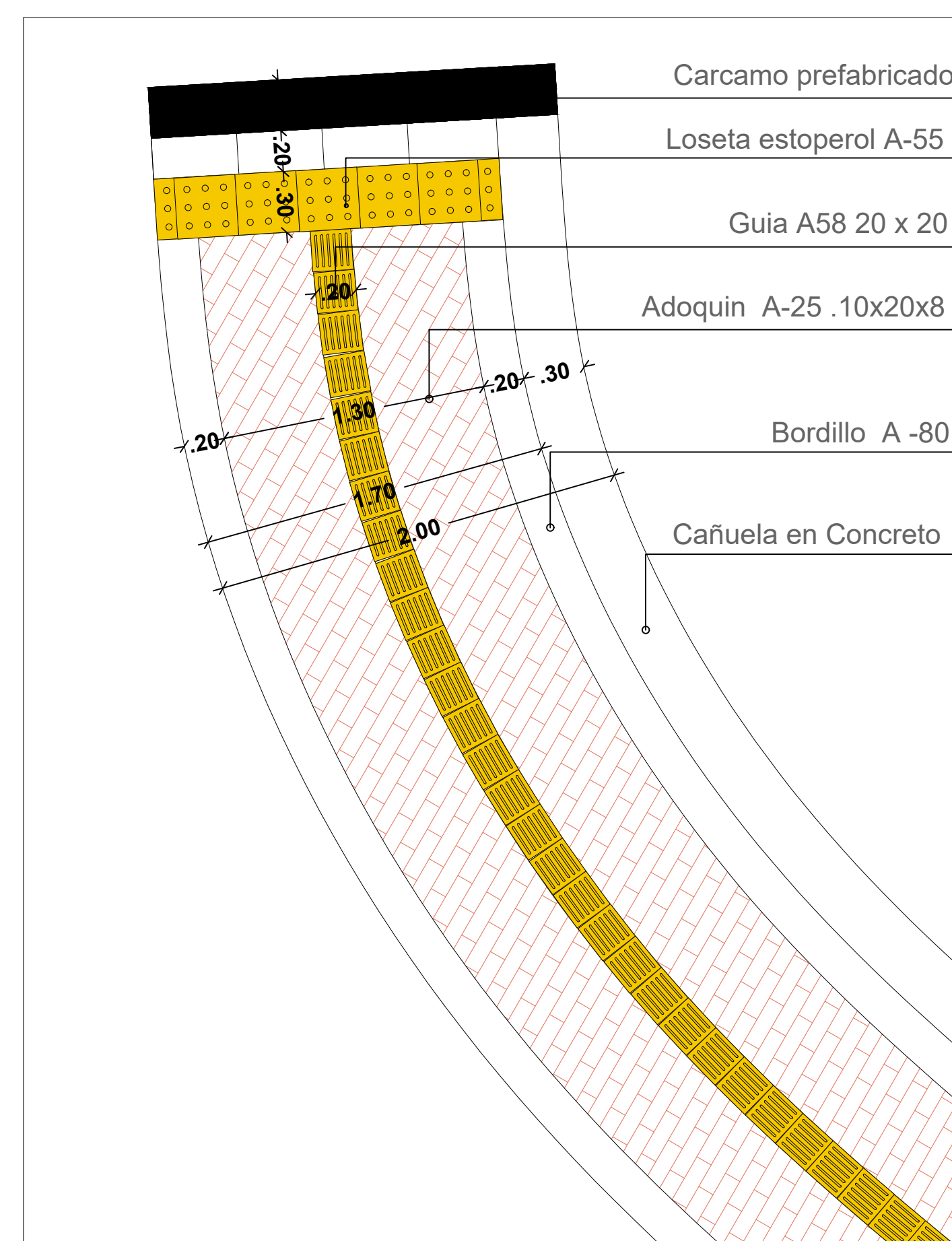
DETALLE EN PLANTA SENDERO
