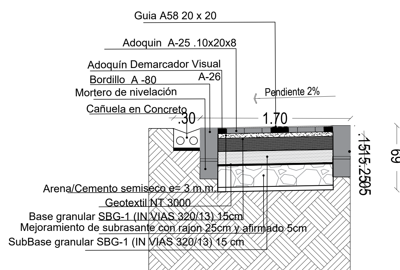
DETALLE PERFIL SENDERO
