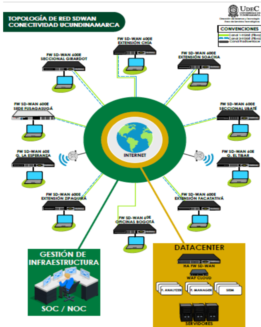
Imagen 1, Topología Deseada - Fuente: Elaboración Propia.
