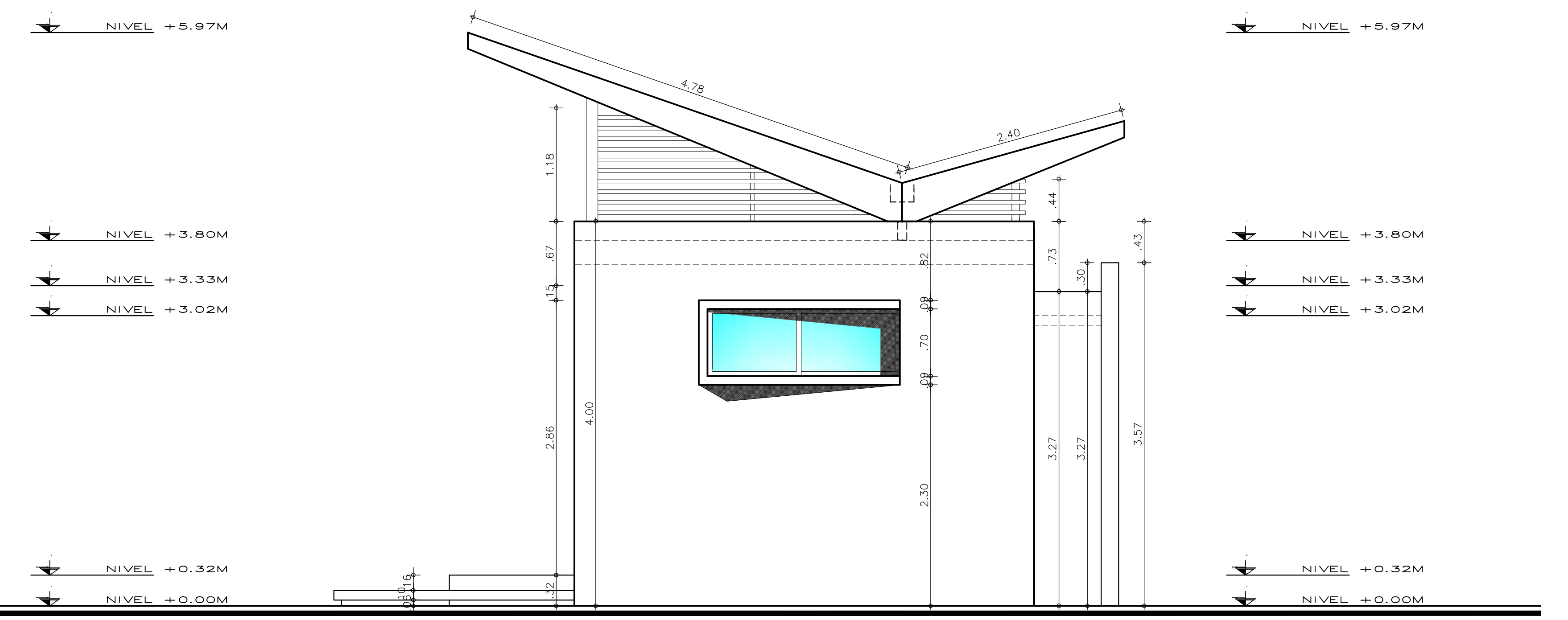
FACHADA LATERAL DERECHA ESC: 1: 50
