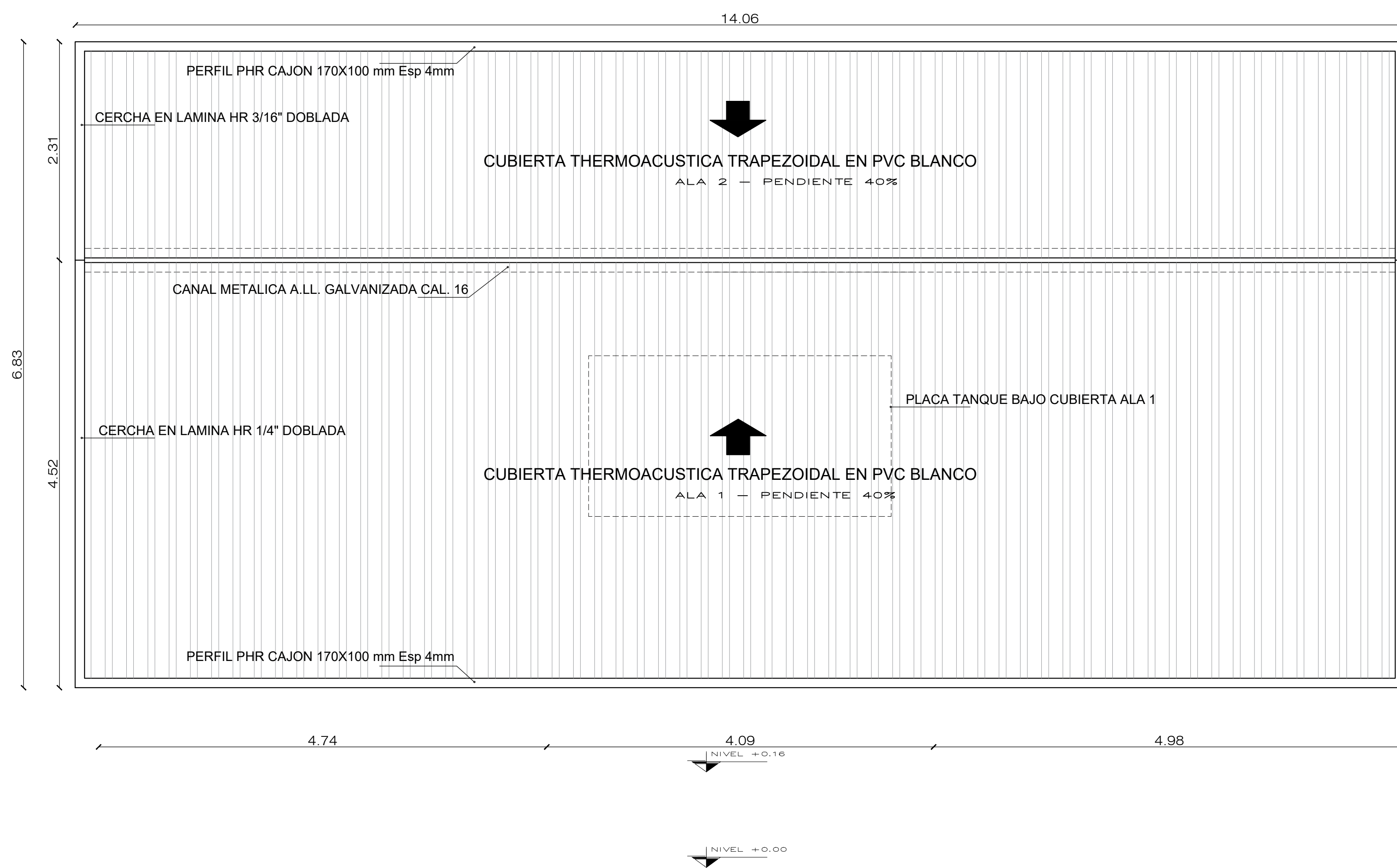
PLANTA CUBIERTAS ESC: 1: 50
