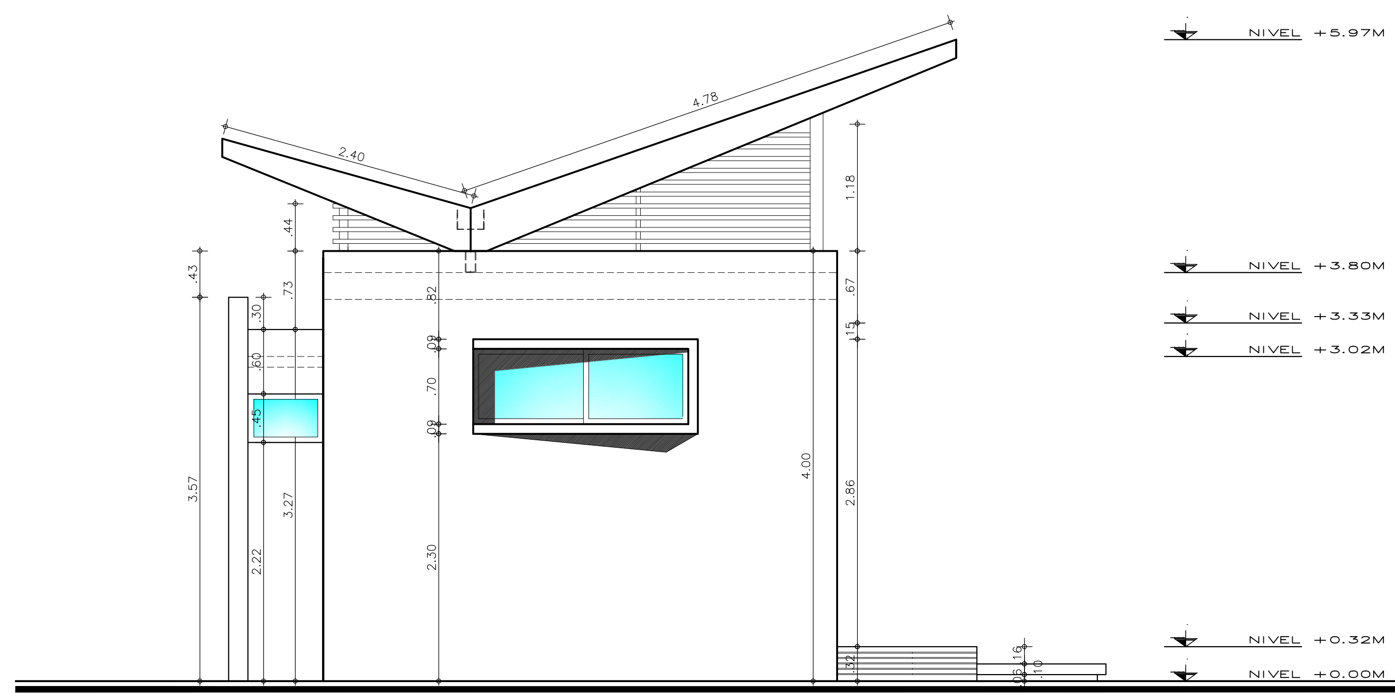
FACHADA LATERAL IZQUIERDA ESC: 1: 50
