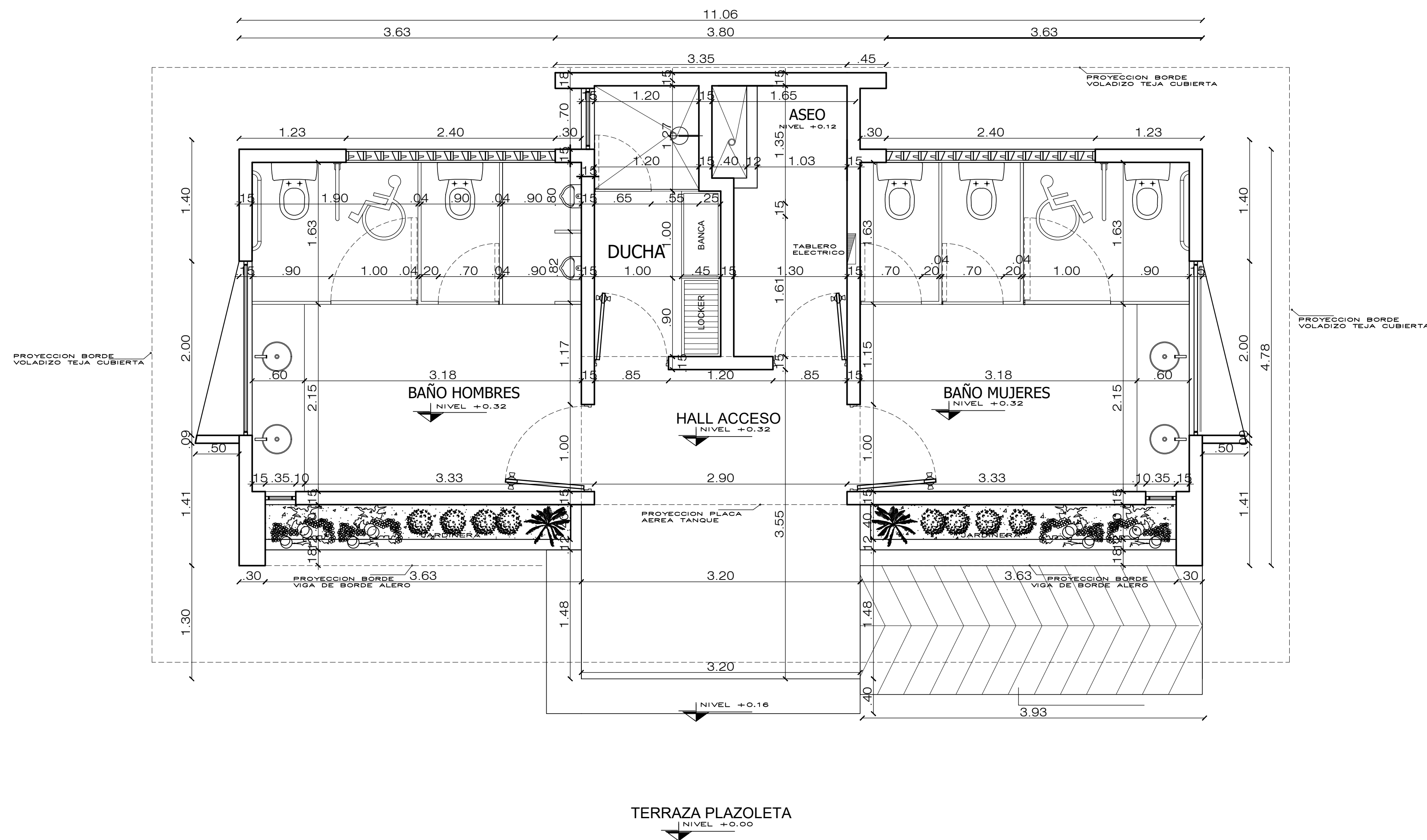
PLANTA ARQUITECTONICA ESC: 1: 50
