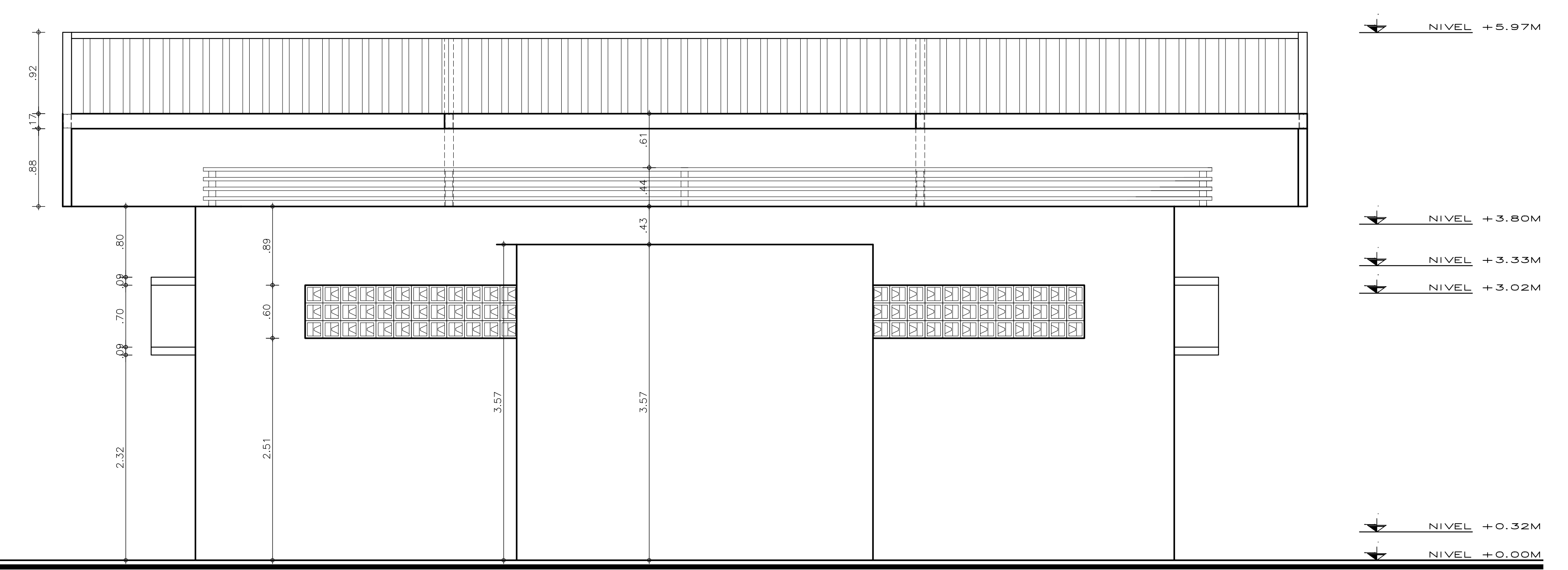
FACHADA POSTERIOR ESC: 1: 50
