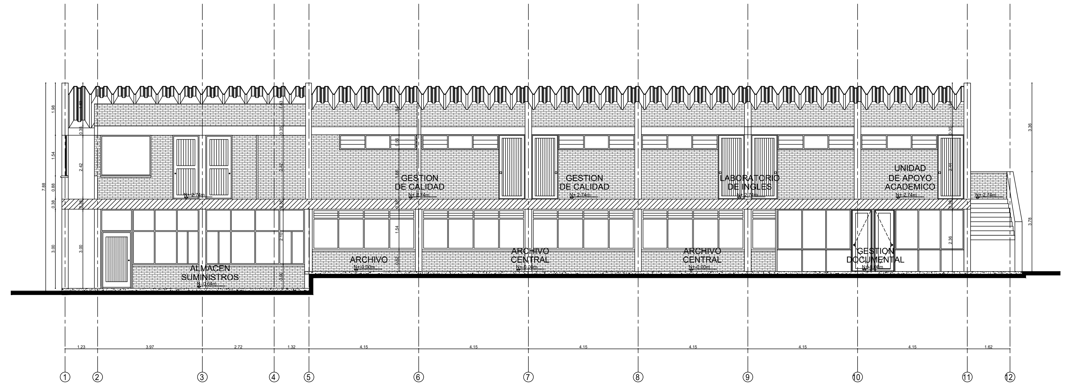
CORTE B - B'
