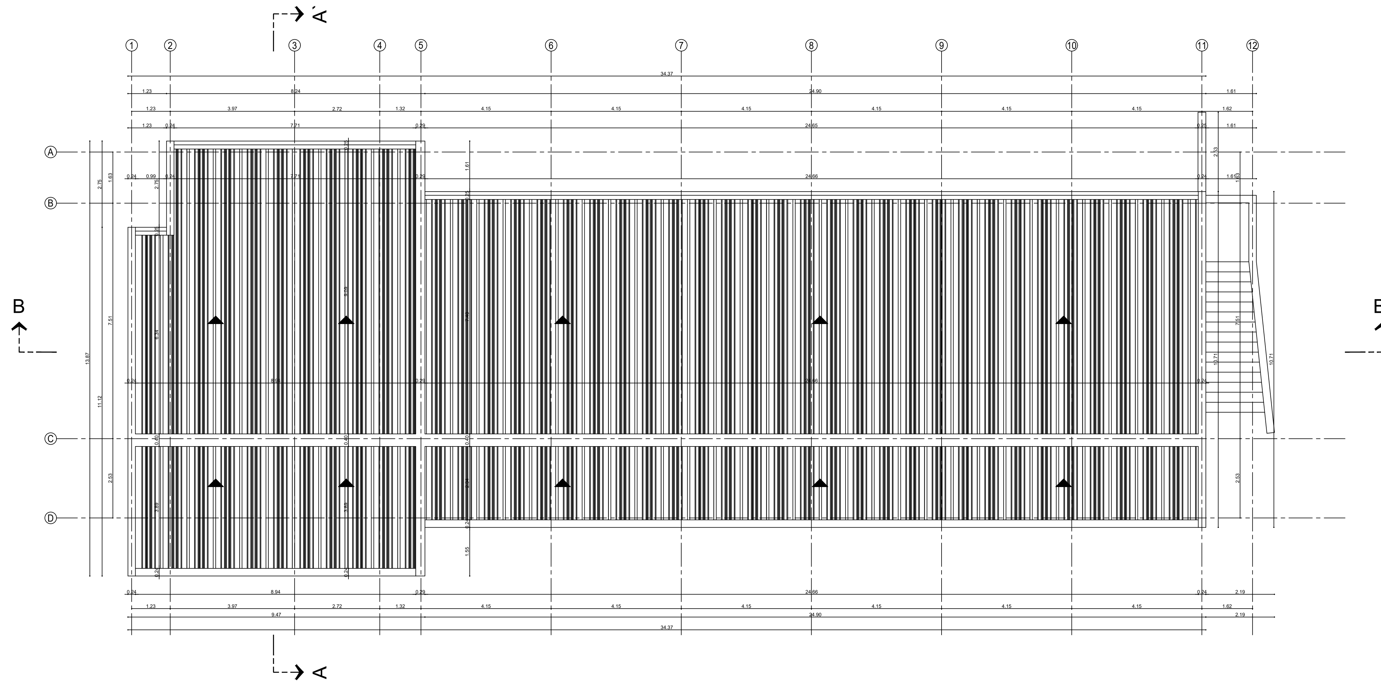
PLANTA DE CUBIERTAS
