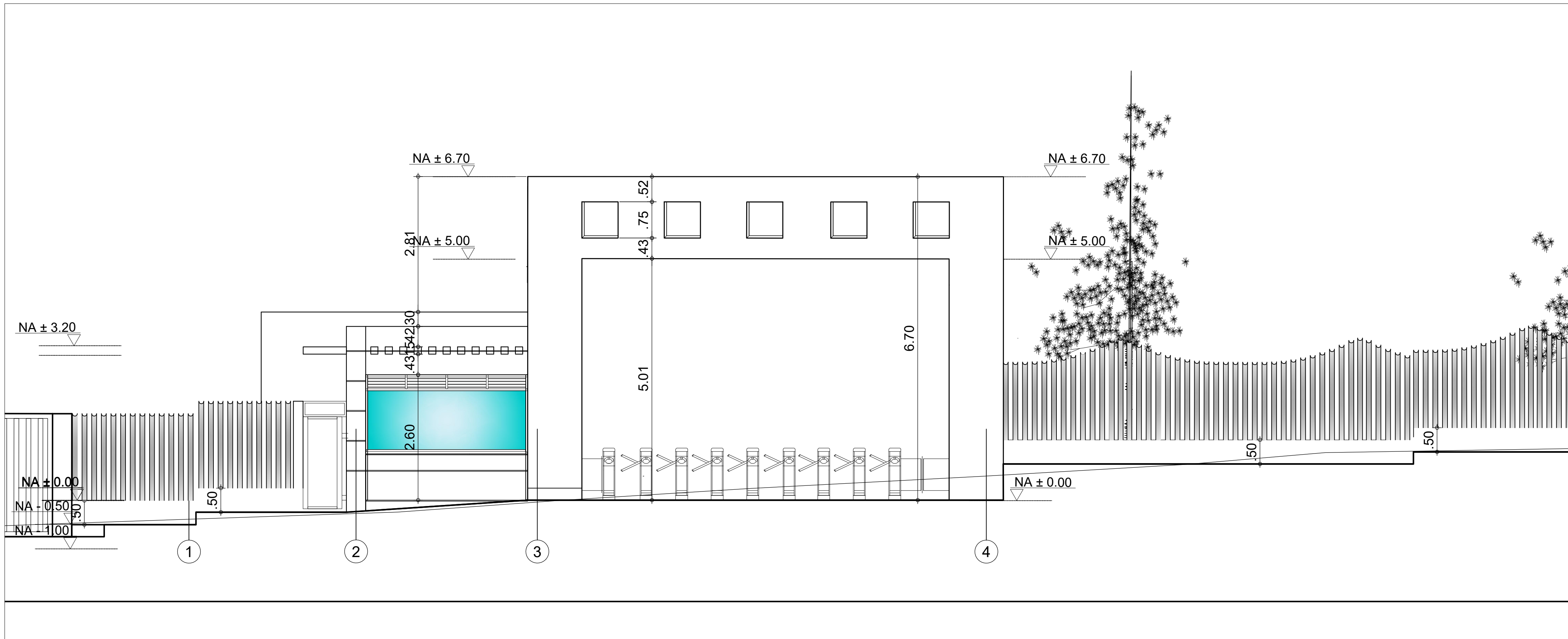
3 FACHADA PUESTO DE CONTROL ACCESO 1:50
