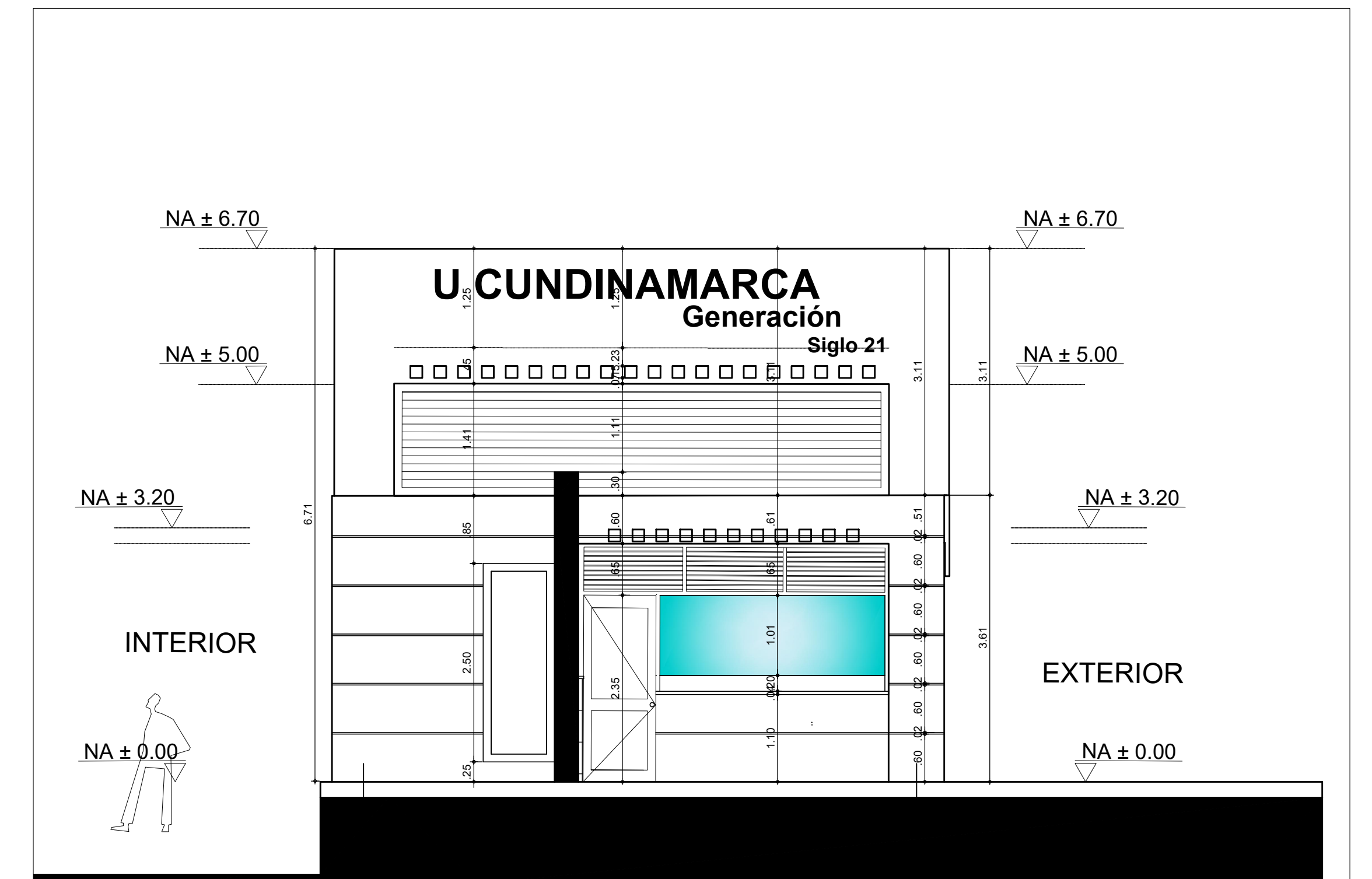
1 FACHADA ACCESO UNIVERSIDAD 1:100
