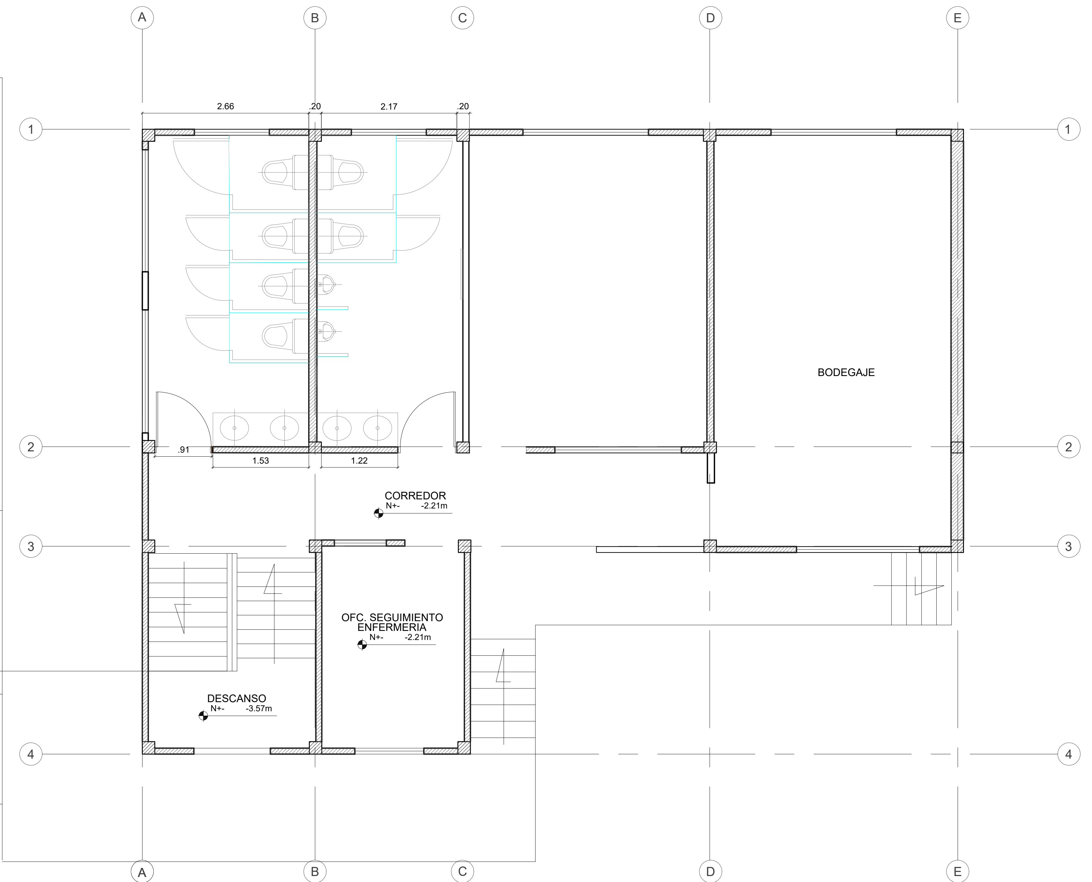
PLANTA SEGUNDO PISO
